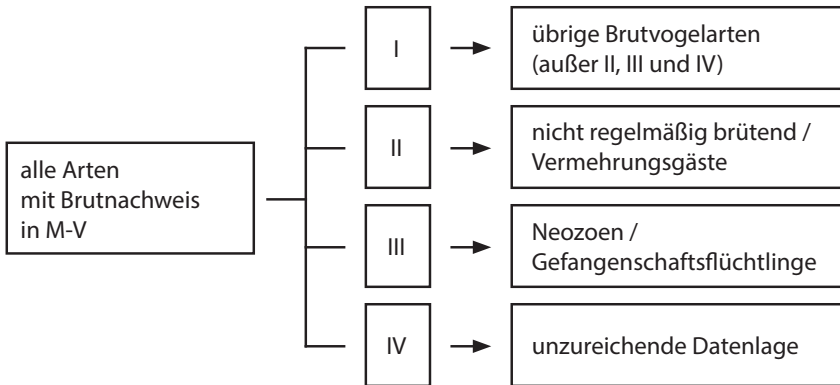
Abb. 1: Zuordnungsschema der Brutvogelarten Mecklenburg-Vorpommerns zu den vier Statuskategorien.
