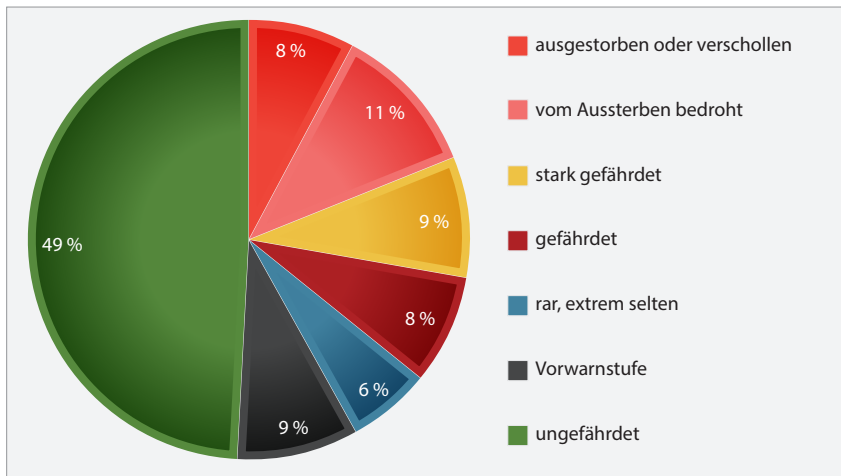
Abb. 10: Gefährdungskategorien der Brutvögel Mecklenburg-Vorpommerns.
