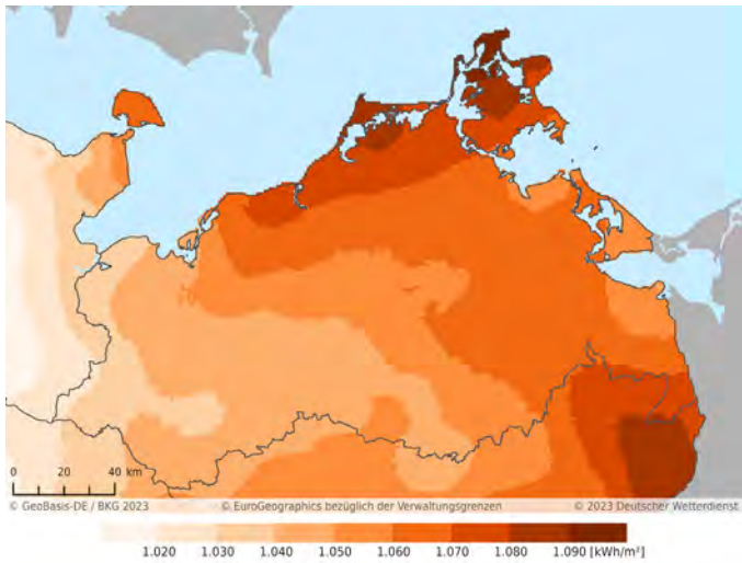
▲ Mittlere Jahressummen der Globalstrahlung [kWh/m 2 ] in Mecklenburg-Vorpommern, basierend auf Bodenmessungen und Satellitendaten der Jahre 1991 – 2020. Auflösung: 1 km x 1 km. Datenbasis: Gebietsmittelwerte des DWD.
