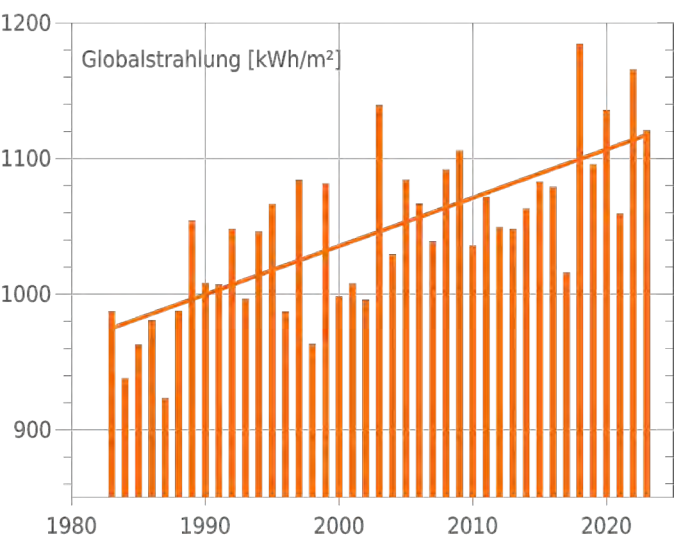
▲ Jahressummen und Trend der Globalstrahlung in Mecklenburg-Vorpommern seit 1983. Datenbasis: Gebietsmittelwerte des DWD.
