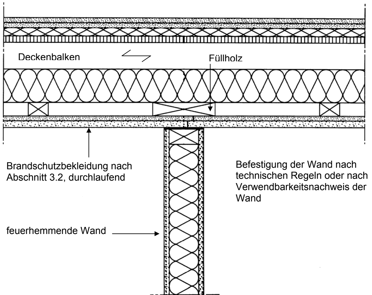
Bild 4 Anschluss einer feuerhemmenden, raumabschließenden, nichttragenden Wand (z. B. Flurwand) an eine Decke nach Abschnitt 3.3.3
