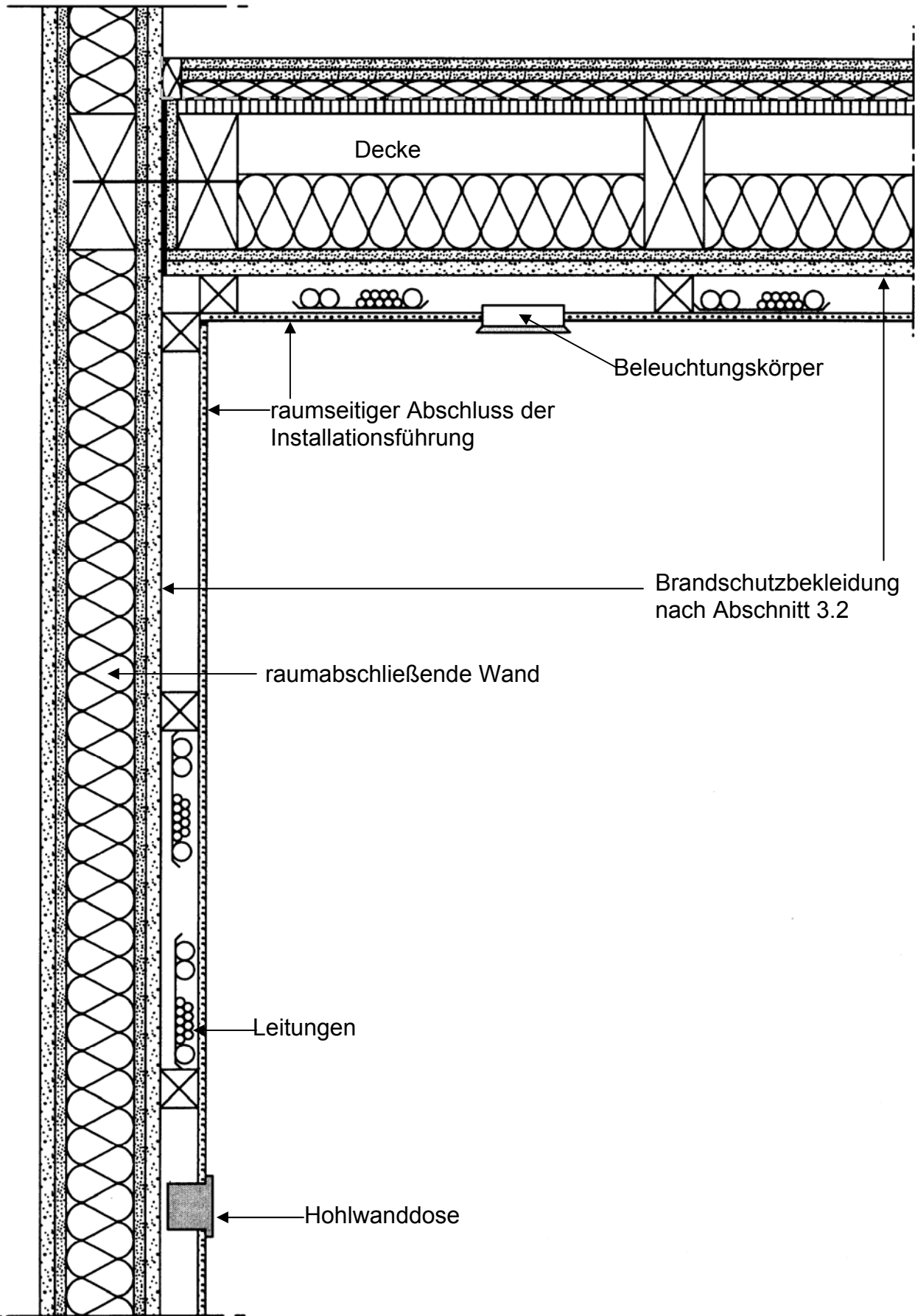
Bild 8 Installationsführung vor der Wand und unterhalb der Decke nach Abschnitt 4.1
