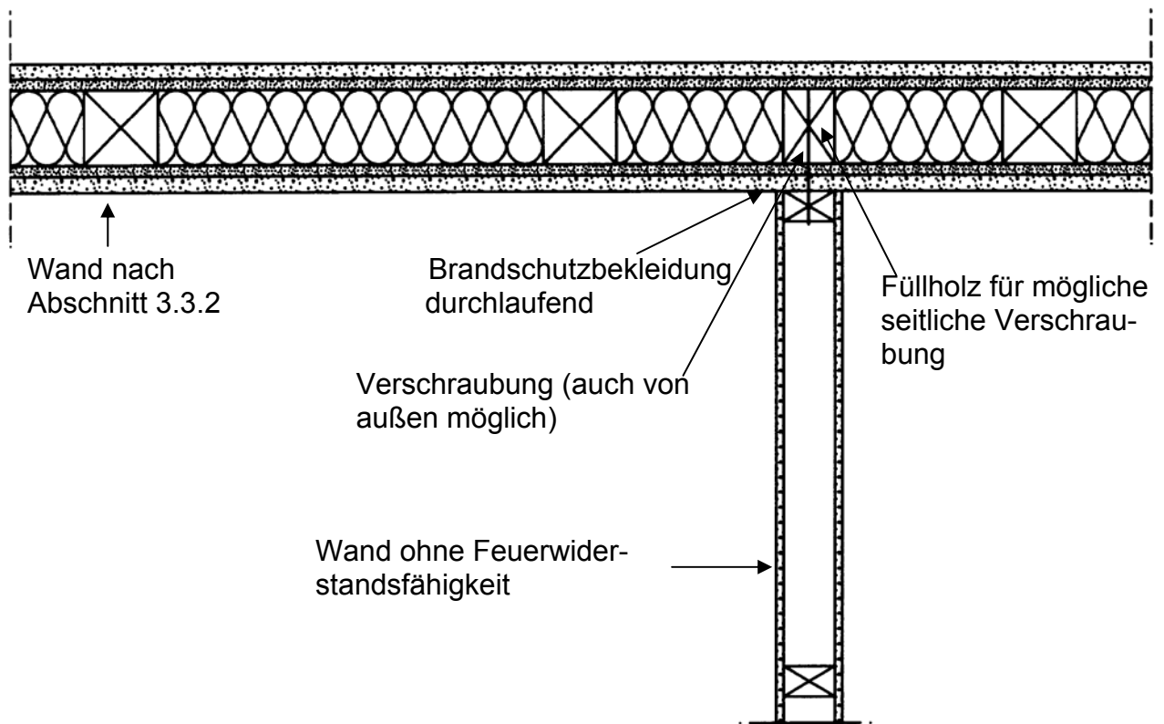
Bild 6 Anschluss einer Wand ohne Feuerwiderstandsfähigkeit an eine Wand nach Abschnitt 3.3.2
