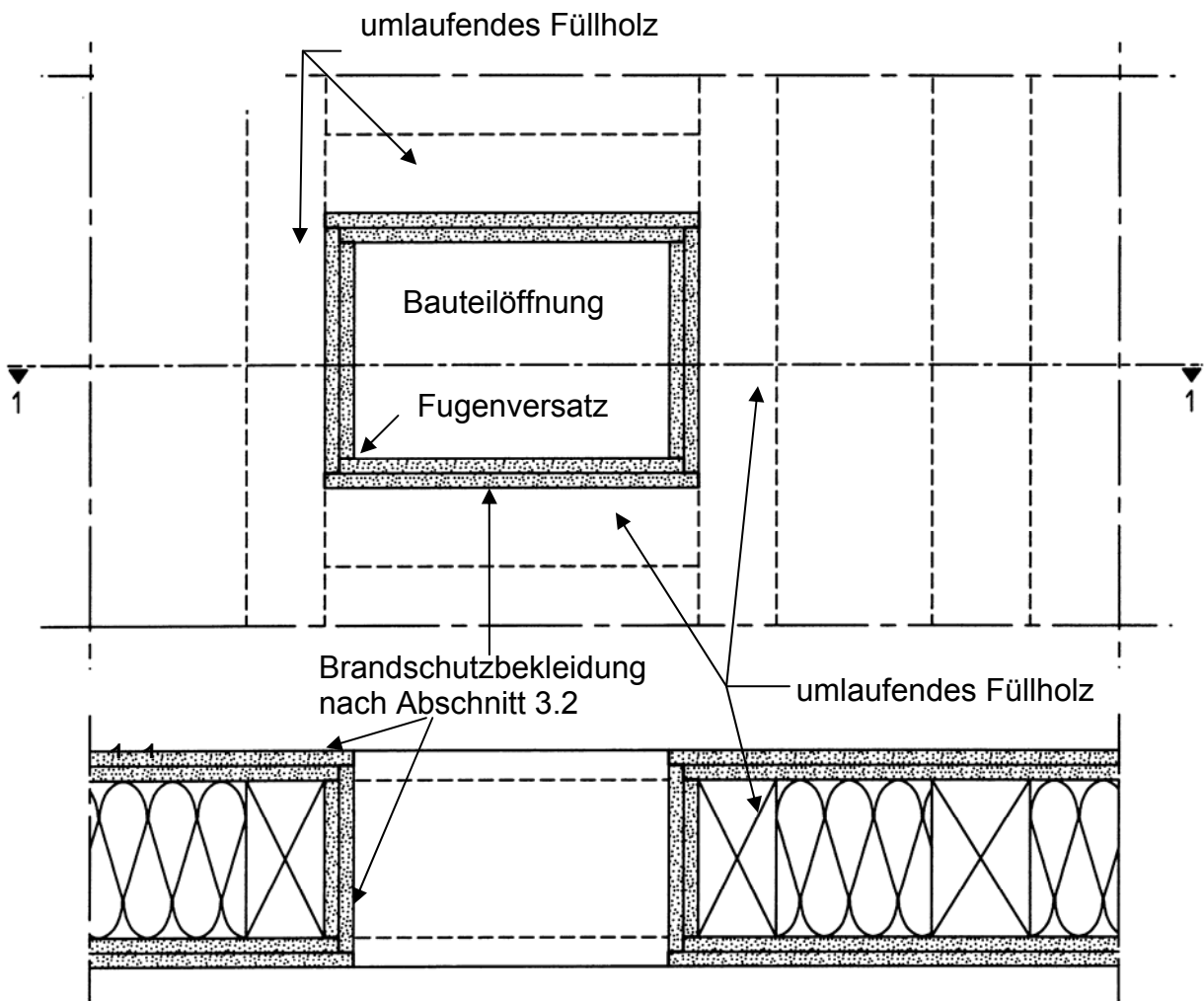
Bild 7 Bauteilöffnung mit Brandschutzbekleidung nach Abschnitt 3.2 zum Einbau von Türen, Fenstern und sonstigen Einbauten nach Abschnitt 3.5 oder zur Durchführung von Schächten, Kanälen und von Installationen nach Abschnitt 4.1 – Darstellung der Ausführung des Fugenversatzes
