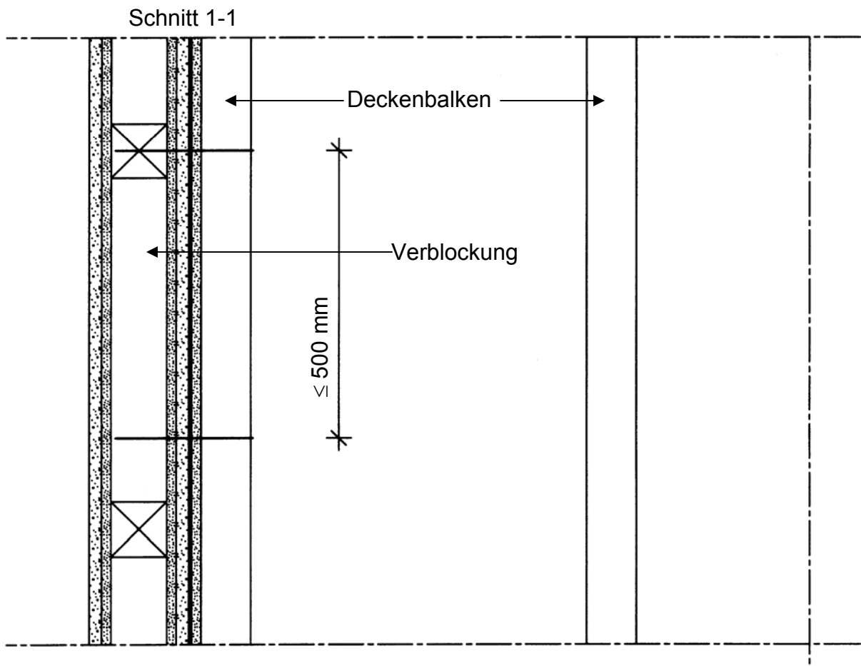
Bild 2 Anschluss Decke nach Abschn. 3.3.3 an durchlaufende raumabschließende Wand nach Abschn. 3.3.2 (Treppenraumwand, Außenwand, auch nichttragend – Spannrichtung der Deckenbalken parallel zur Wand)
