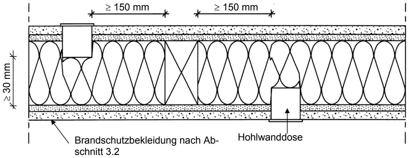
Bild 9 Einbau einzelner Hohlwanddosen nach Abschnitt 4.2, zweiter Absatz
