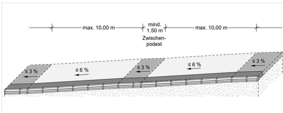
Abb. II 9 – maximale Längsneigung von Gehwegen bzw. gemeinsamen Geh- und Radwegen
