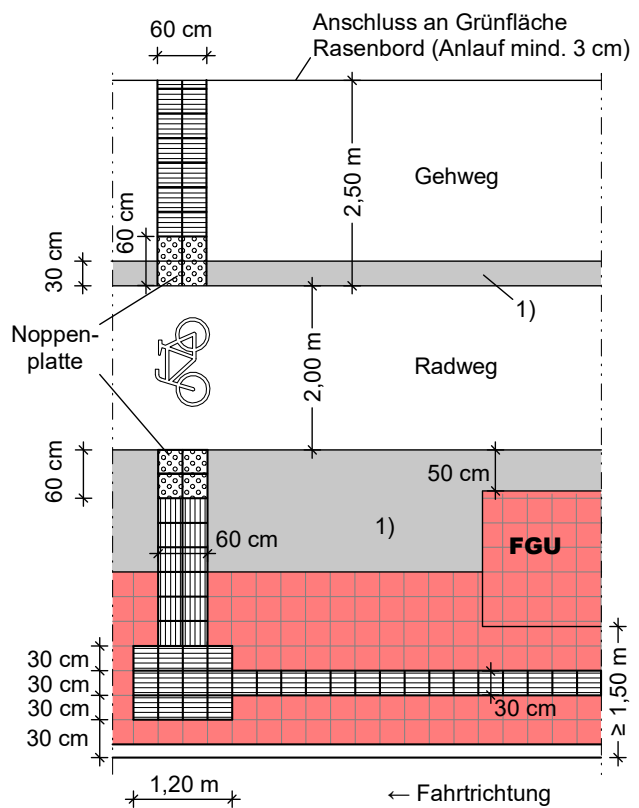
2. mit angrenzendem Radweg- und Gehweganbindung
