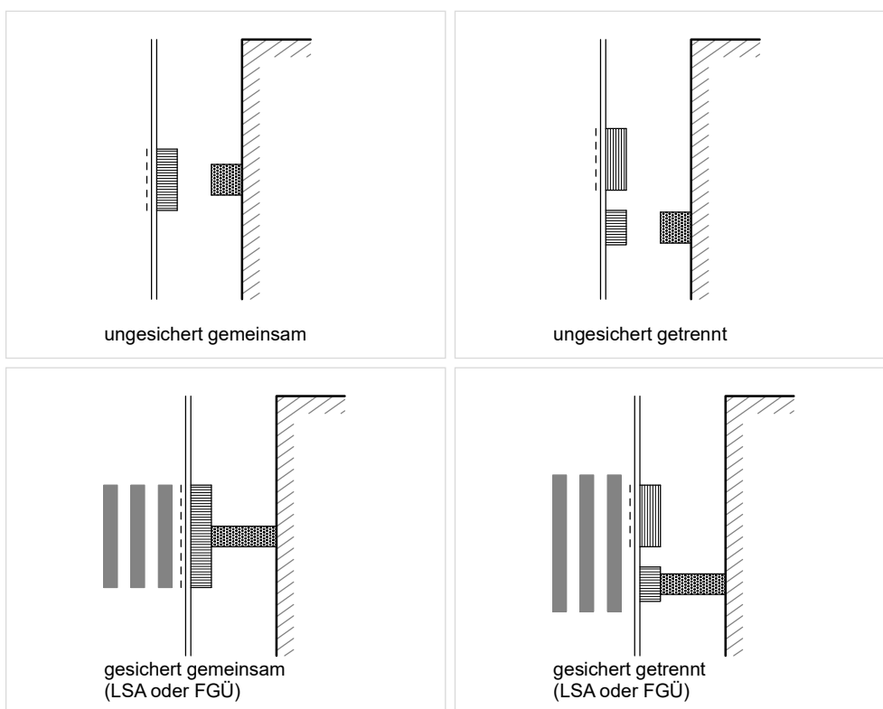
Abb. IV 2 – Formen von Überquerungsstellen
