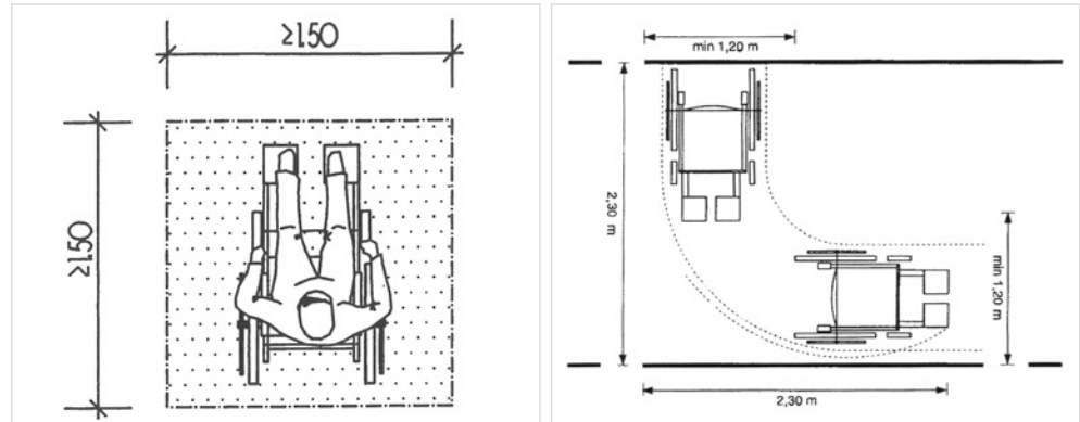
Abb. II 6 – Flächenbedarf für Rollstuhlnutzung bei Drehung bzw. Kurvenfahrt
