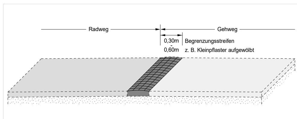
Abb. II 17 – Begrenzungsstreifen aufgewölbt
