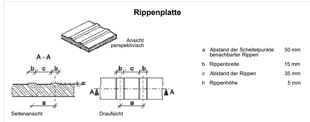
Abb. II 26 – Rippenplatte
