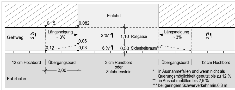
Abb. II 12 – Gehweg mit Teilung des Quergefälles
