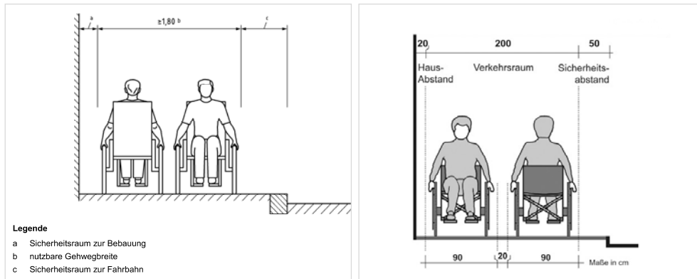
Abb. II 4 – Raumbedarf für die Begegnung zweier Rollstühle
