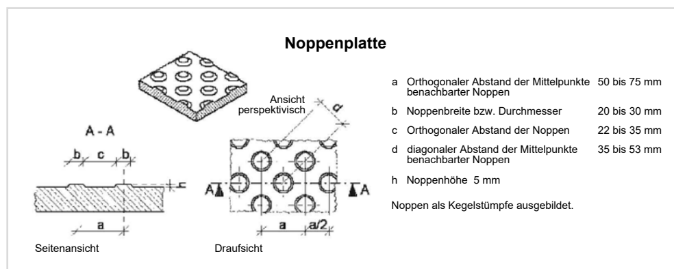
Abb. II 32 – Noppenplatte
