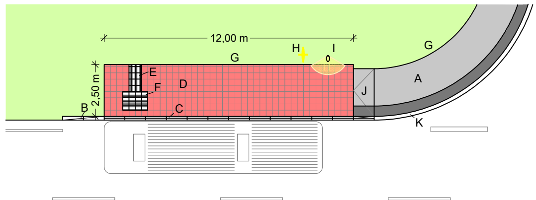
Bushaltestelle mit Wegeanbindung (außerorts)
