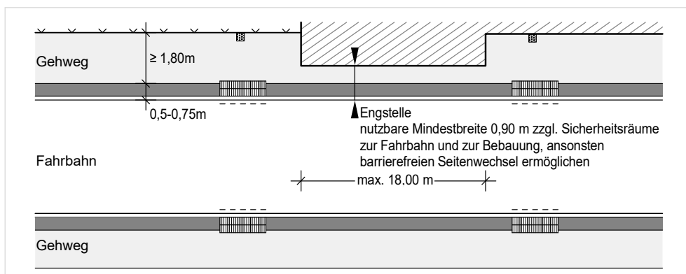
Abb. II 5 – Engstelle mit Umwegung
