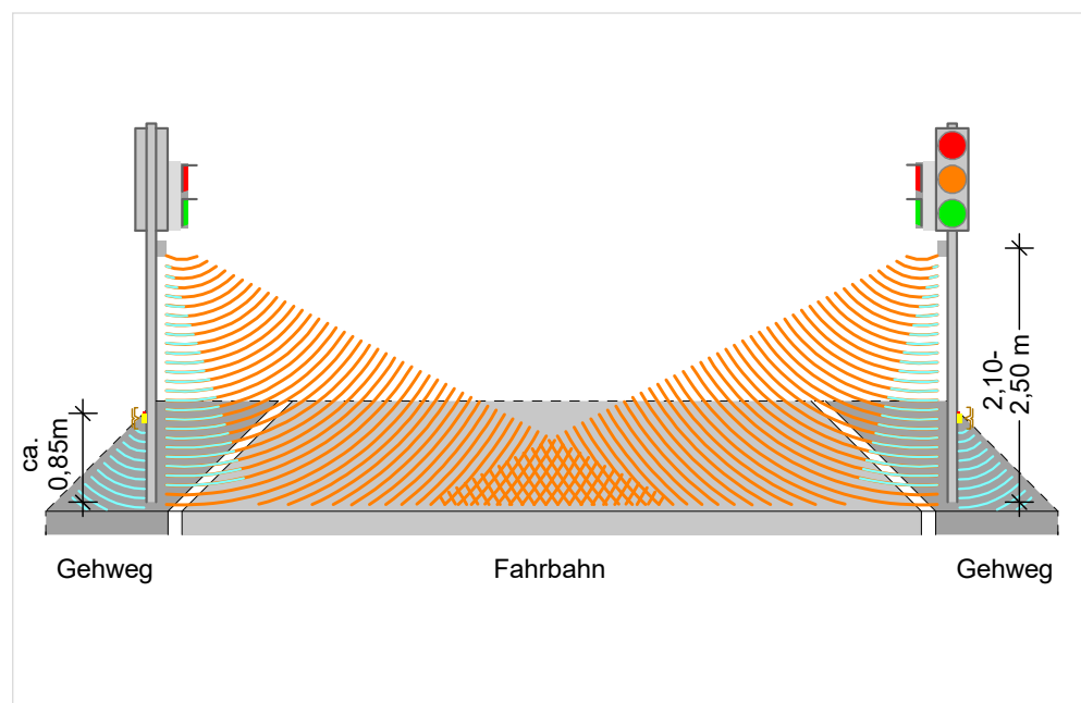
Abb. II 19 – Schallausrichtung (optimal) für Orientierungs- und Freigabesignal
