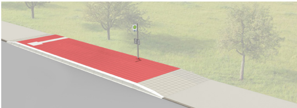
Abb. II 46 – Beispiel für Bushaltestelle Kategorie D
