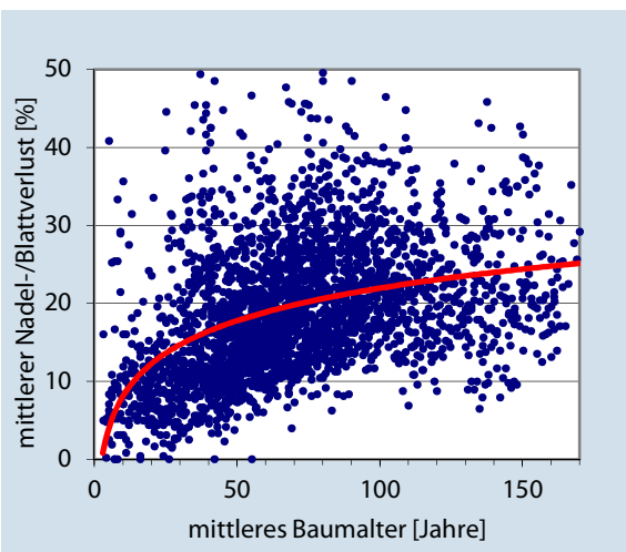
Abb. 10: Mittlerer Nadel-/Blattverlust in Abhängigkeit vom mittleren Baumalter der Stichprobenpunkte der Waldzustandserhebung. Rote Linie: Trend der Nadel-/Blattverluste über dem Alter.
