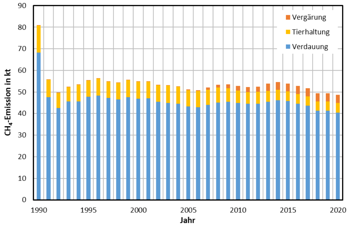
Abbildung 9: CH 4 -Emissionen der Landwirtschaft von 1990 bis 2020
