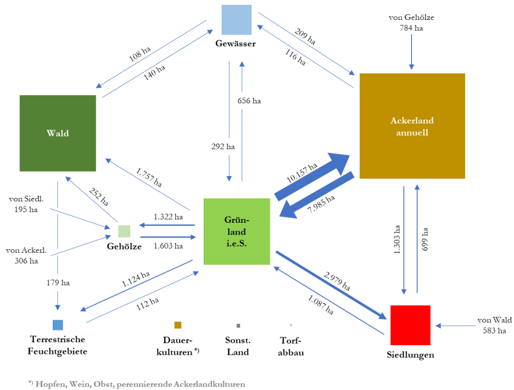
Abbildung 15: Landnutzungsänderungen 2017 (ab 100 ha, schematisch) 23
