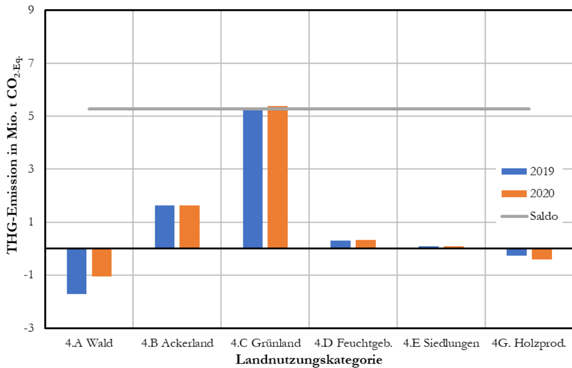
Abbildung 11: Treibhausgasemissionen aus LULUCF 2019 und 2020 nach Kategorien
