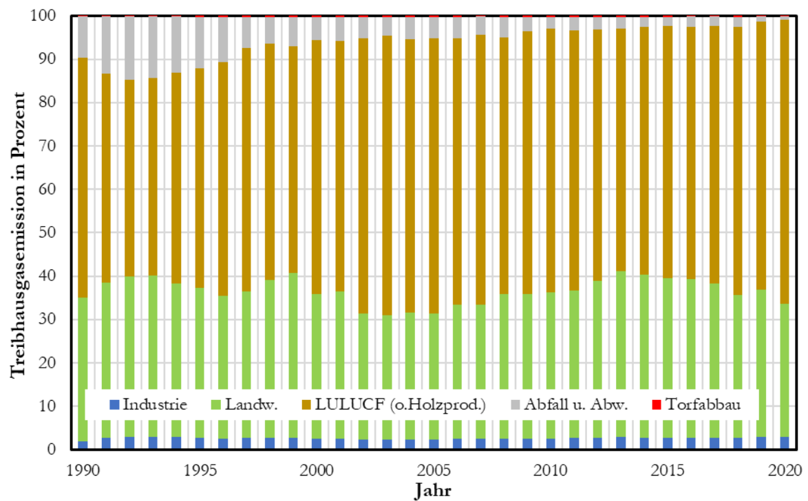
Abbildung 2: Struktur der nicht energiebedingten Treibhausgasemissionen von 1990 bis 2020
