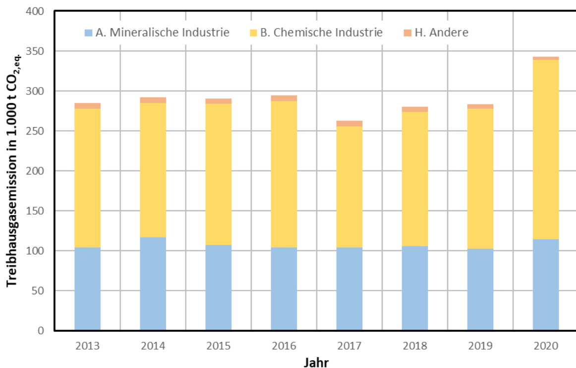
Abbildung 4: Treibhausgasemissionen der Industrie nach Branchen von 2013 bis 2020 15
