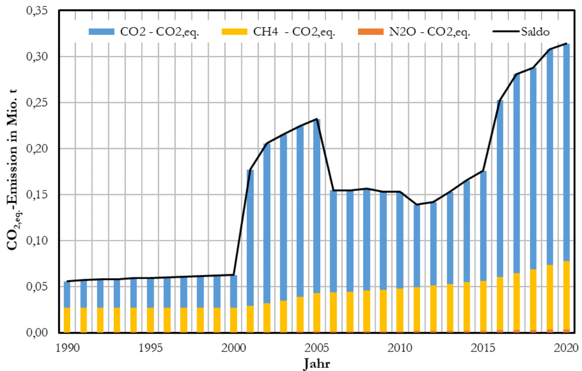
Abbildung 21: Treibhausgasemissionen aus LULUCF-Feuchtgebiete von 1990 bis 2020
