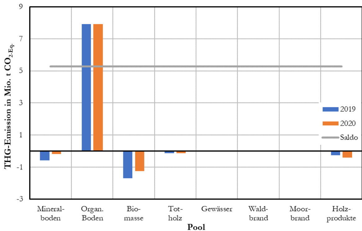
Abbildung 12: Treibhausgasemissionen aus LULUCF 2019 und 2020 nach Pools
