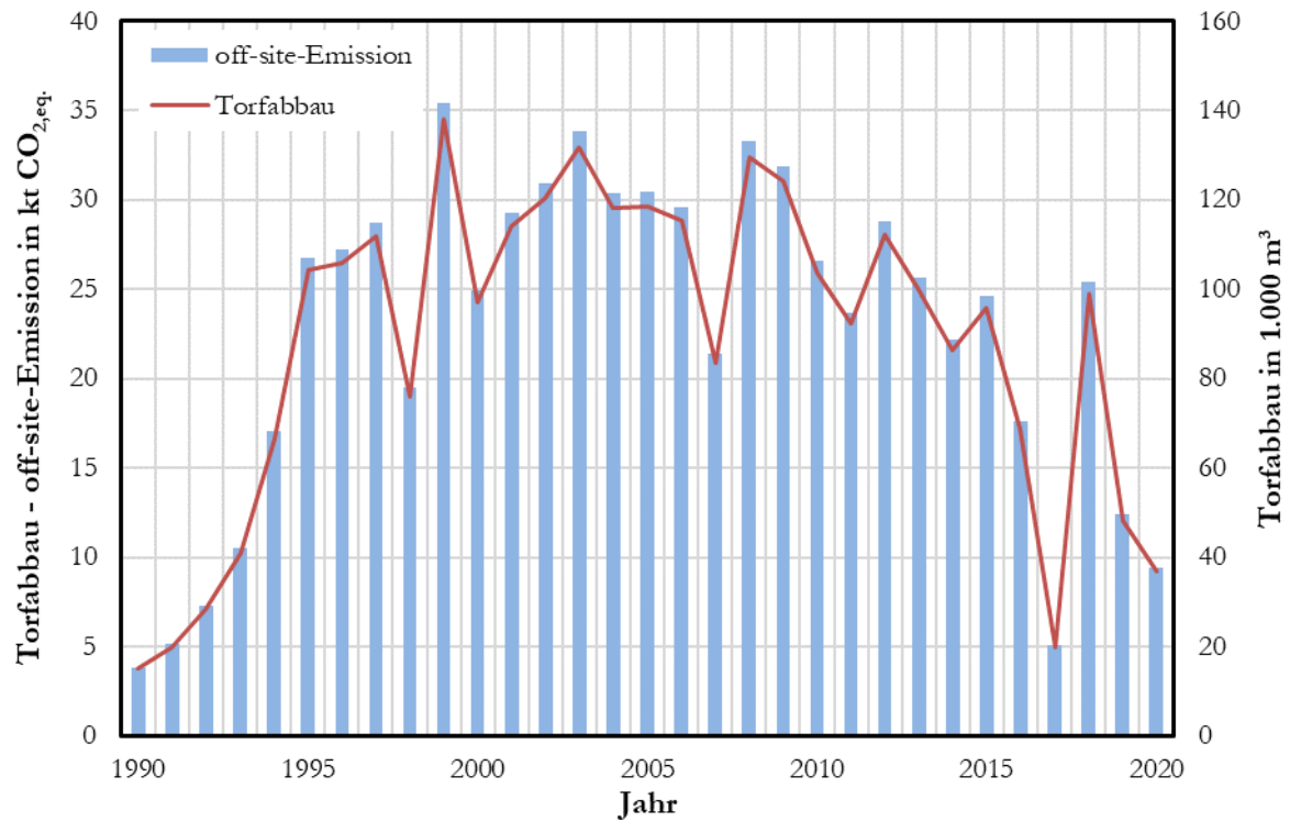
Abbildung 20: off-site-Treibhausgasemissionen aus dem Torfabbau von 1990 bis 2020
