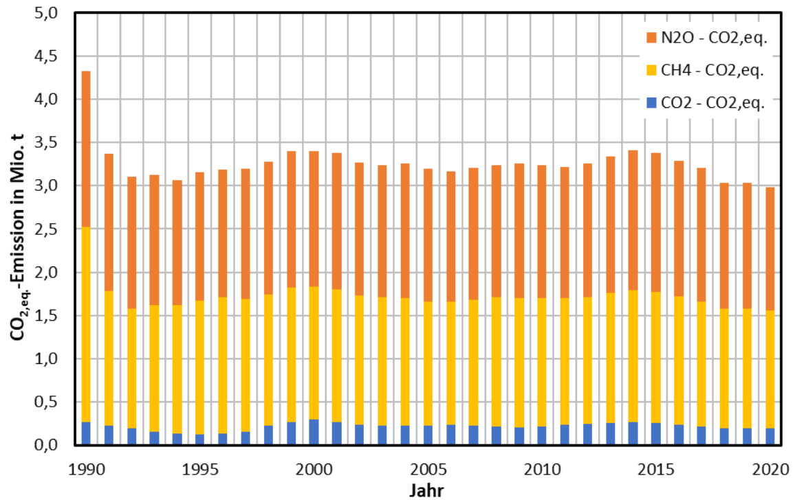
Abbildung 6: Treibhausgasemissionen der Landwirtschaft nach Gasen von 1990 bis 2020
