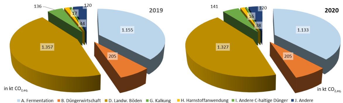
Abbildung 5: Treibhausgasemissionen der Landwirtschaft 2019 und 2020
