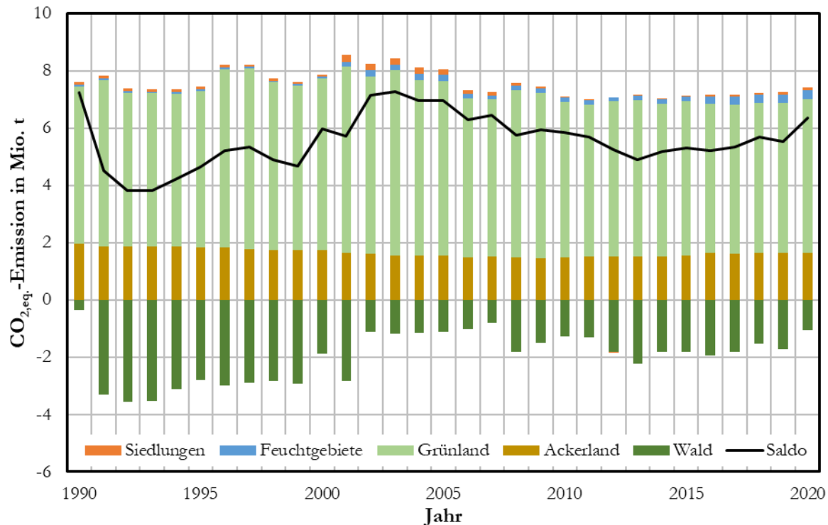
Abbildung 14: Treibhausgasemissionen aus LULUCF 1990 bis 2020 (ohne Holzprodukte)
