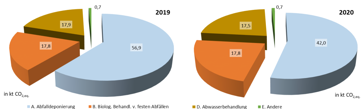
Abbildung 23: Treibhausgasemissionen Abfall und Abwasser 2019 und 2020
