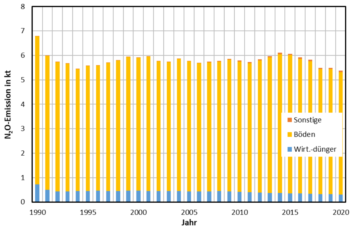
Abbildung 10: N 2 O-Emissionen der Landwirtschaft von 1990 bis 2020
