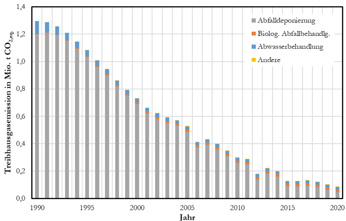
Abbildung 24: Treibhausgasemissionen Abfall und Abwasser von 1990 bis 2020
