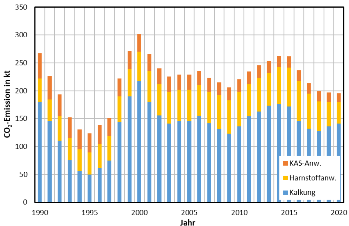
Abbildung 8: CO 2 -Emissionen der Landwirtschaft von 1990 bis 2020
