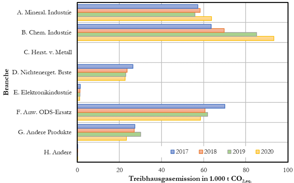
Abbildung 3: Treibhausgasemissionen der Industrie nach Branchen 2017 bis 2020 12
