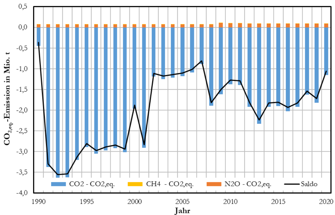
Abbildung 17: Treibhausgasemissionen aus LULUCF-Wald von 1990 bis 2020
