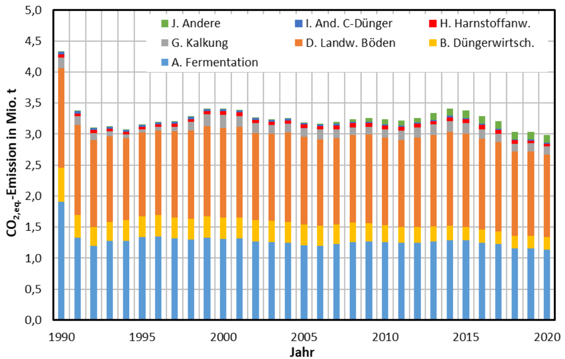
Abbildung 7: Treibhausgasemissionen der Landwirtschaft nach Bereichen von 1990 bis 2020
