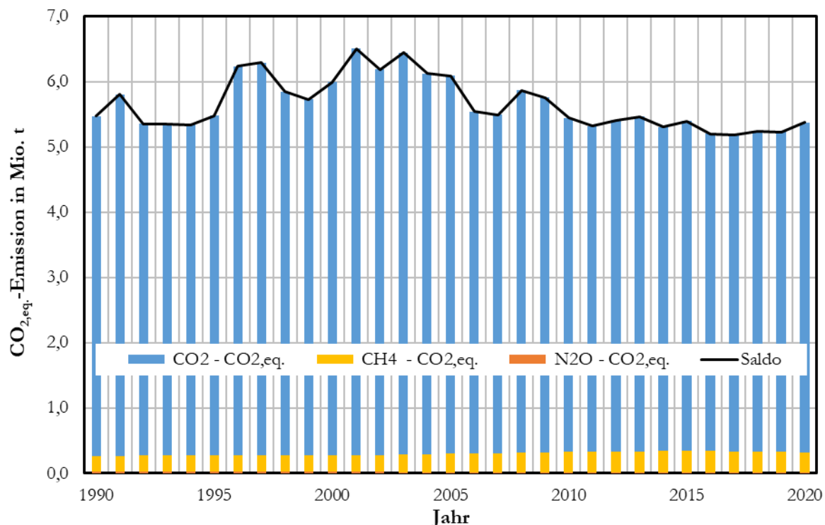
Abbildung 19: Treibhausgasemissionen aus LULUCF-Grünland von 1990 bis 2020
