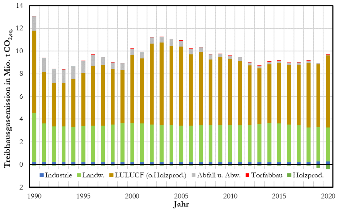
Abbildung 1: Nicht energiebedingte Treibhausgasemissionen von 1990 bis 2020
