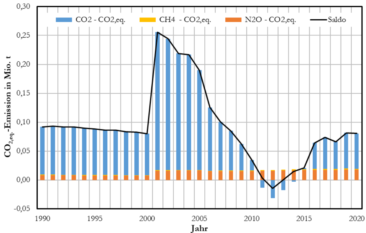
Abbildung 22: Treibhausgasemissionen aus LULUCF-Siedlungen von 1990 bis 2020
