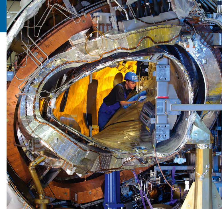
Wendelstein 7-X in Greifswald während der Aufbauphase © MPI für Plasmaphysik, Wolfgang Filser
